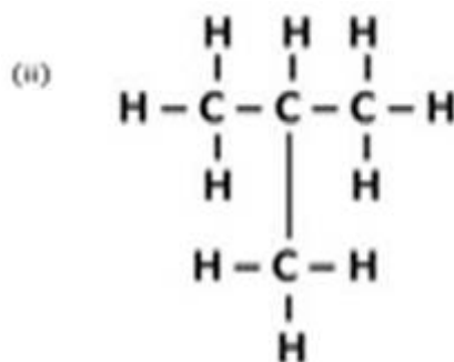
Iso - butane
