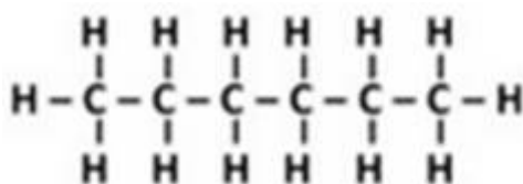
n - hexane
